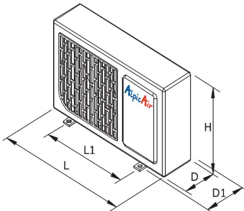
AOU-35HPR1
